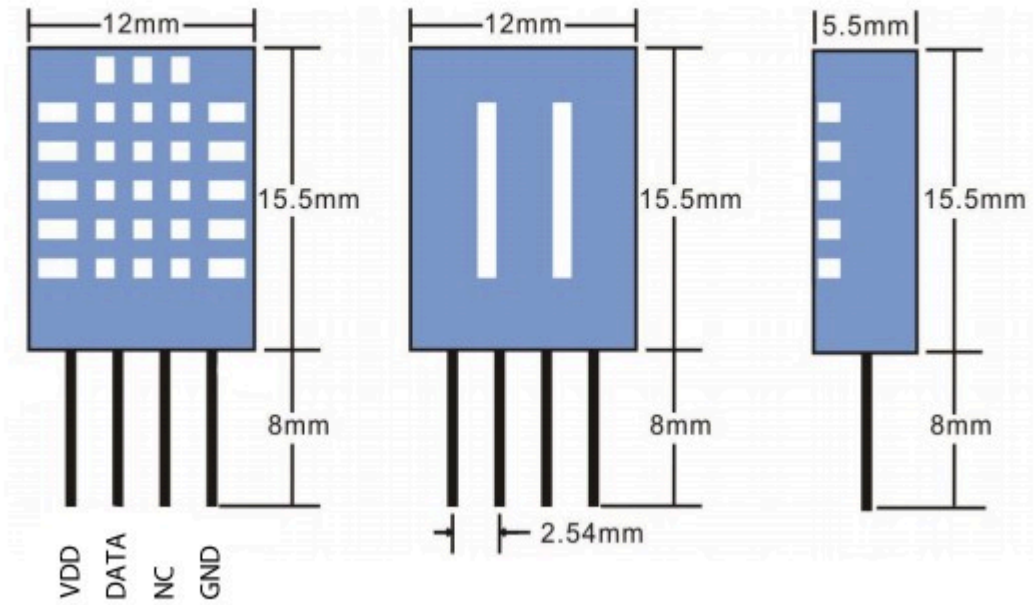
Dimensões e Pinagem Sensor DHT11
