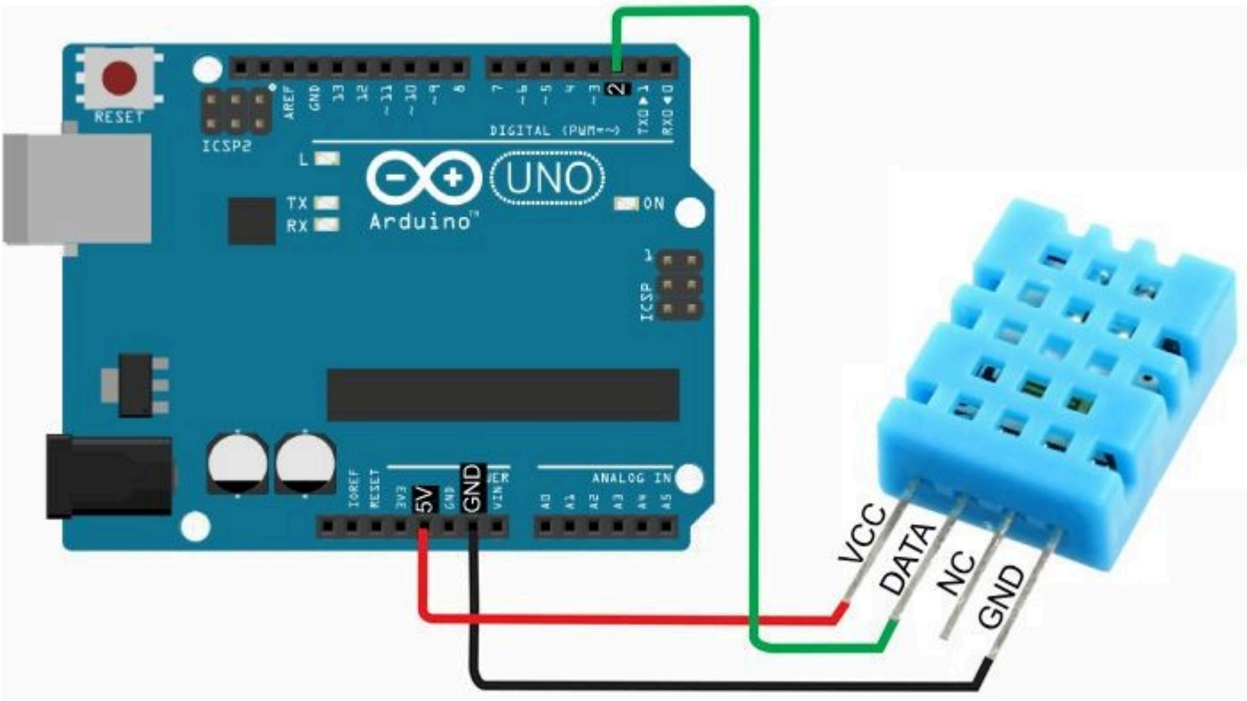
Conexão Sensor DHT11 com Arduino
